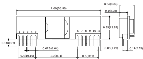
<SIP TYPE>
