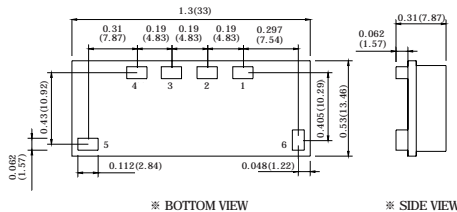
<SMT TYPE>
